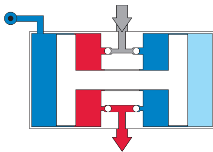
動作原理 GPLV 2
